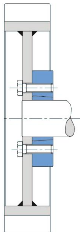
Befestigung des KN22-Drivesrades mit einer Klemmnabe KN22
